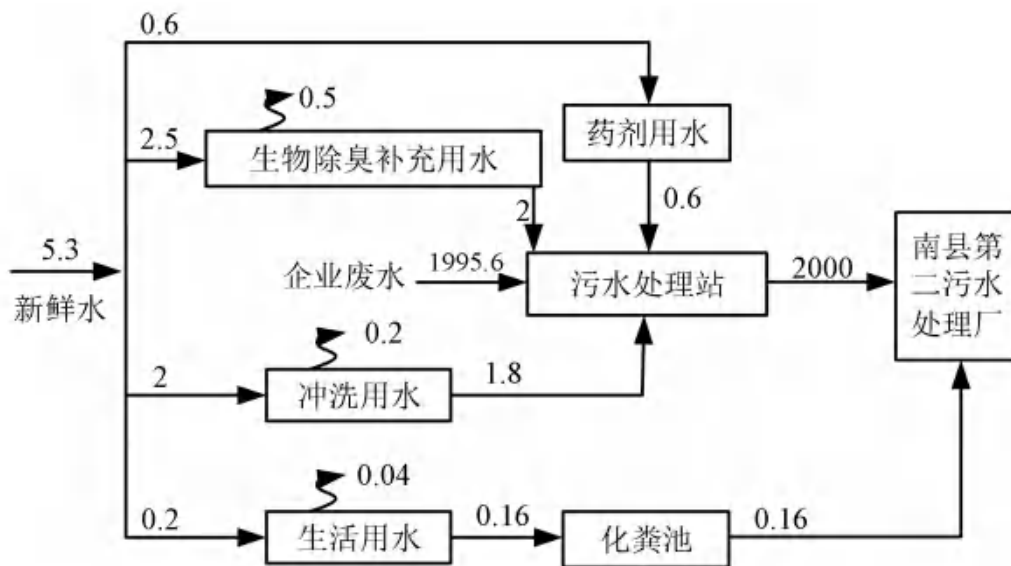
图 3.1-3 项目水平衡图 ( \text{m}^3/\text{d} )
