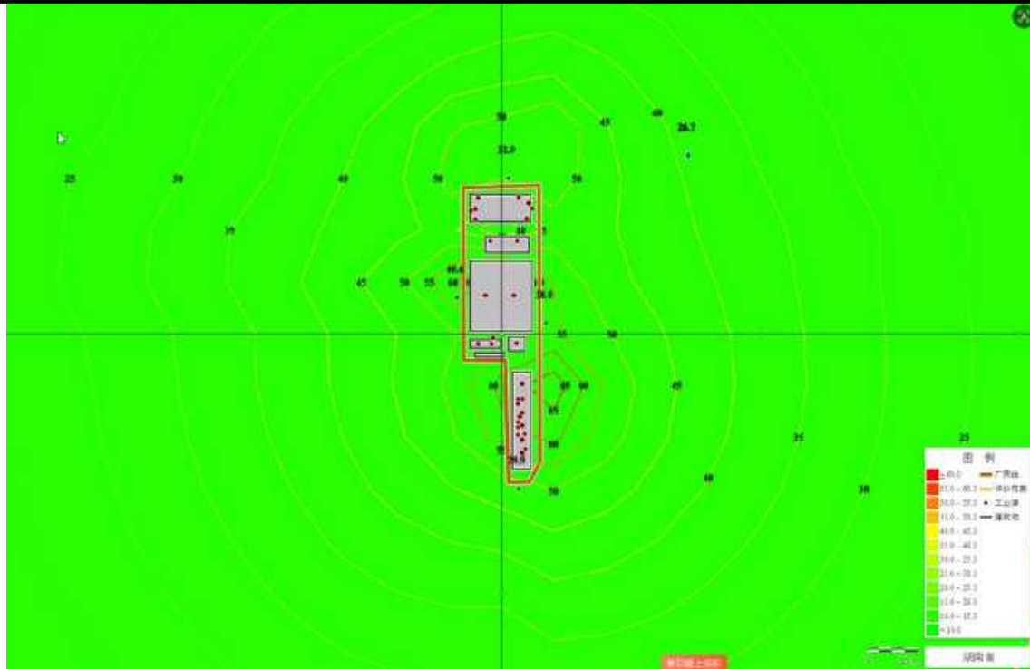
图 5.8-1 项目厂界噪声预测结果图
