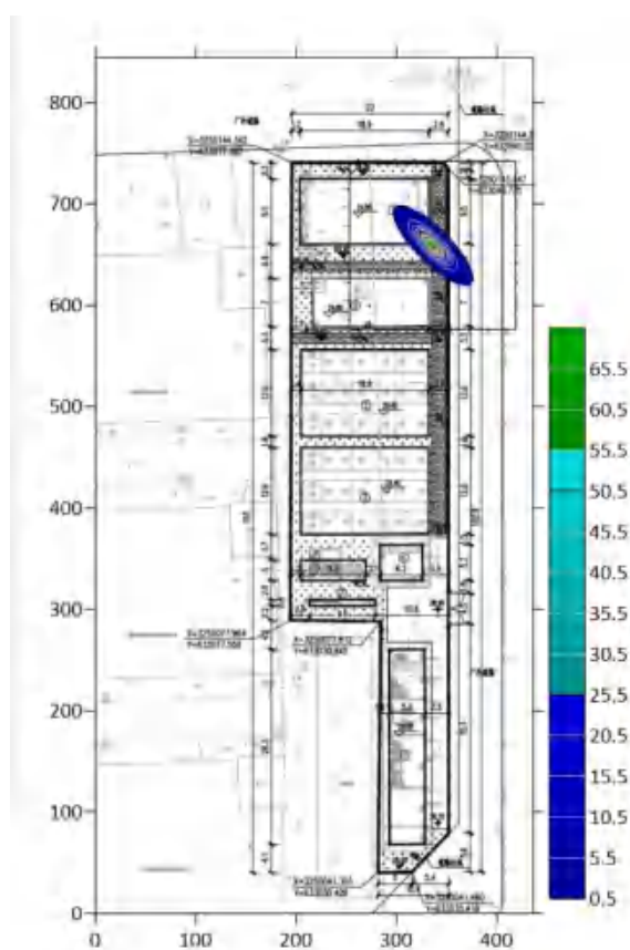
图5.7-2 1000天氨氮迁移距离
