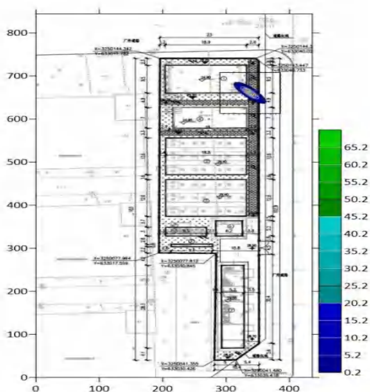
图5.7-1 100天氨氮迁移距离
