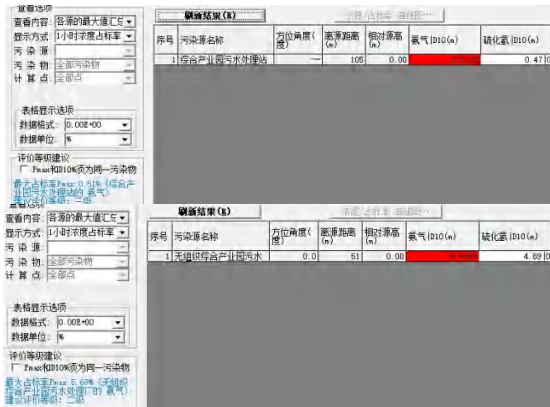
图 5.6-1 各源 1 小时浓度最大占标率结果
