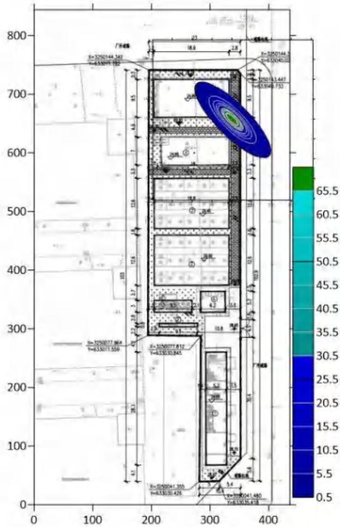
图5.7-3 5000天氨氮迁移距离
