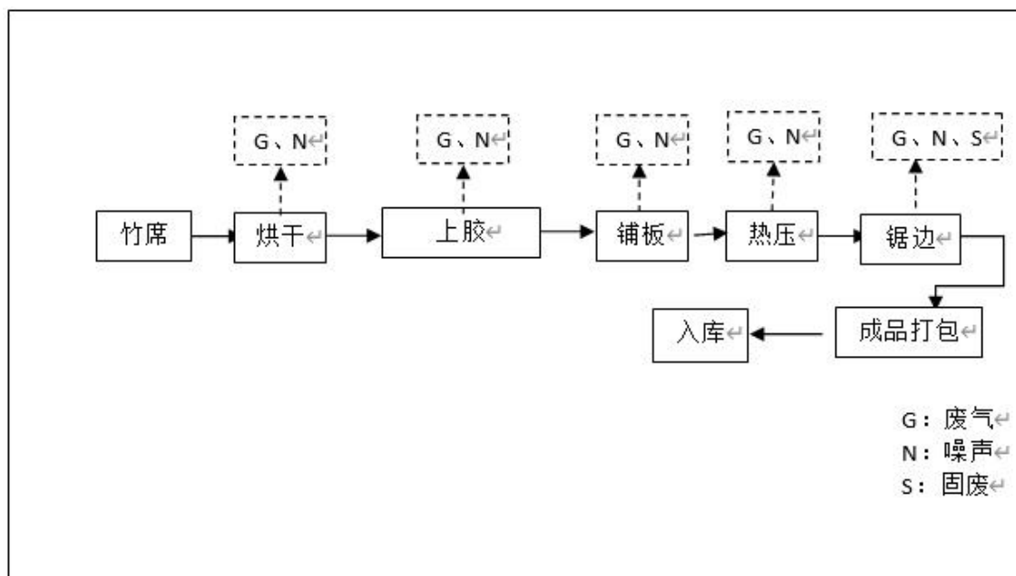
图 2-3 竹胶板生产工艺流程图
