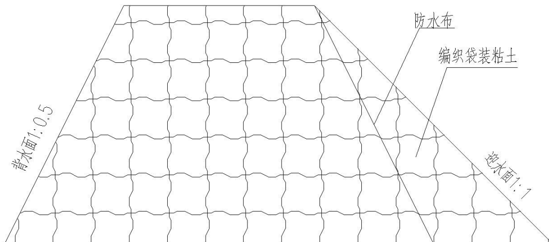
图 3.3-7 围堰断面大样图
