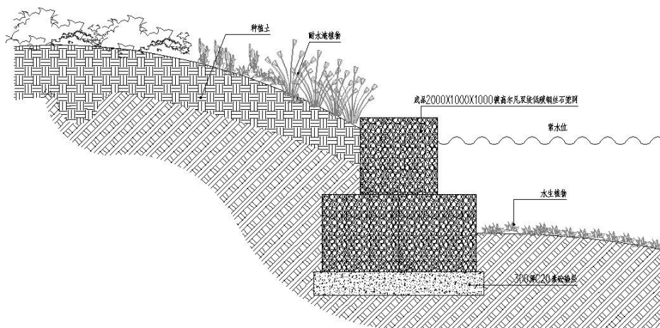
高位岛迎水面大样图
