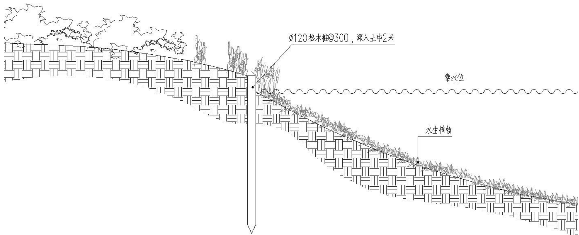
高位岛背水面大样图
