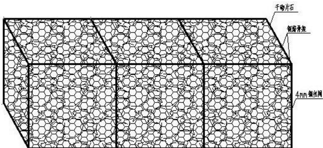
图3.3-3 格宾石笼示意图
