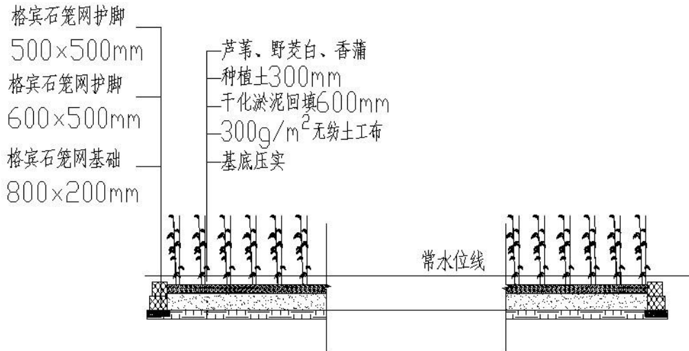
图3.3-5 河滨湿地中位岛大样图
