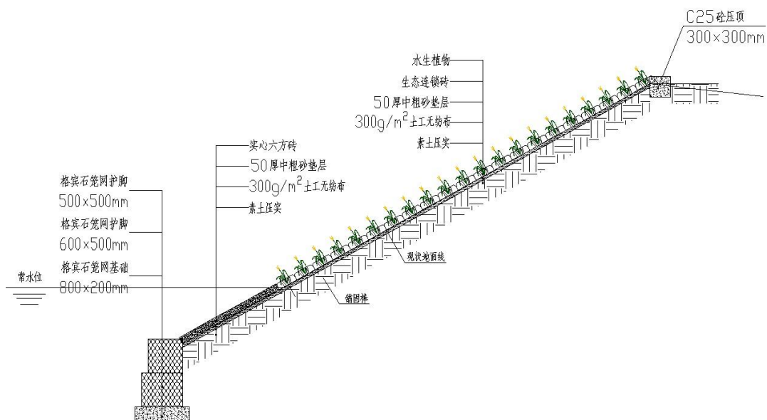
图 3.3-1 生态护岸断面大样图
