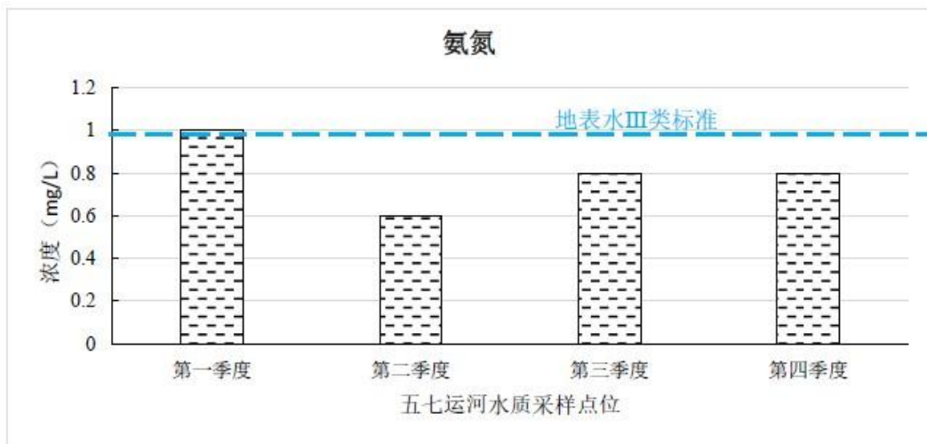
图3.1-5 五七运河氨氮浓度变化
