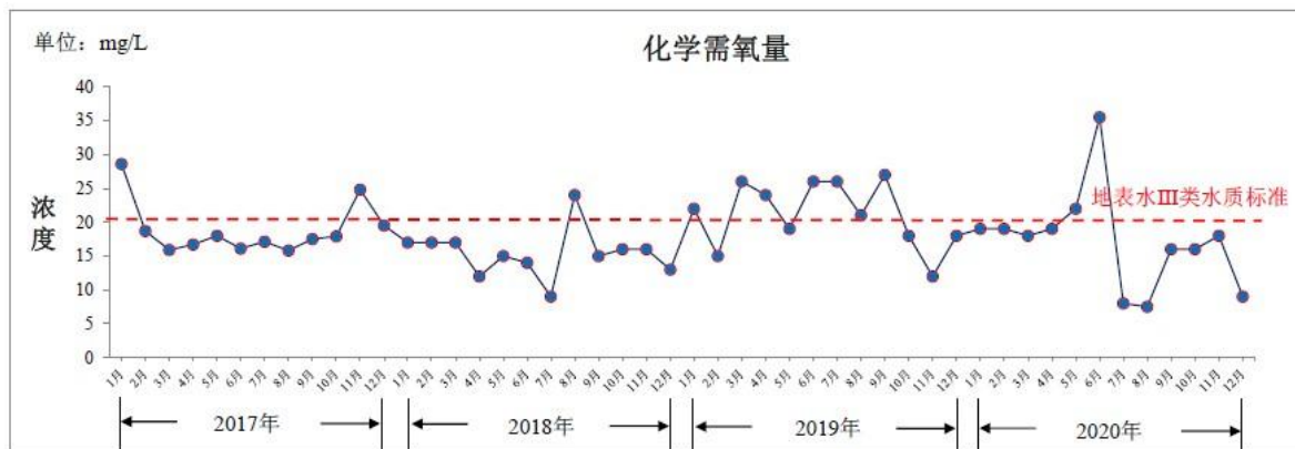
图3.1-1大通湖段面2017-2020年化学需氧量月均浓度变化
