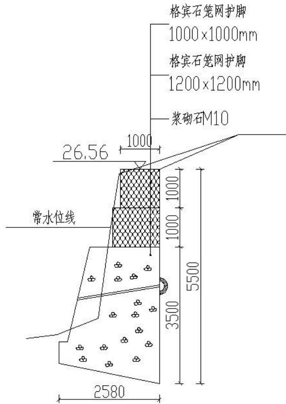
图3.3-4 浆砌石挡土墙+格宾石笼护坡大样图
