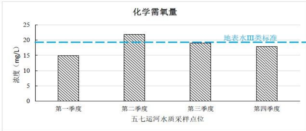
图3.1-4 五七运河化学需氧量浓度变化
