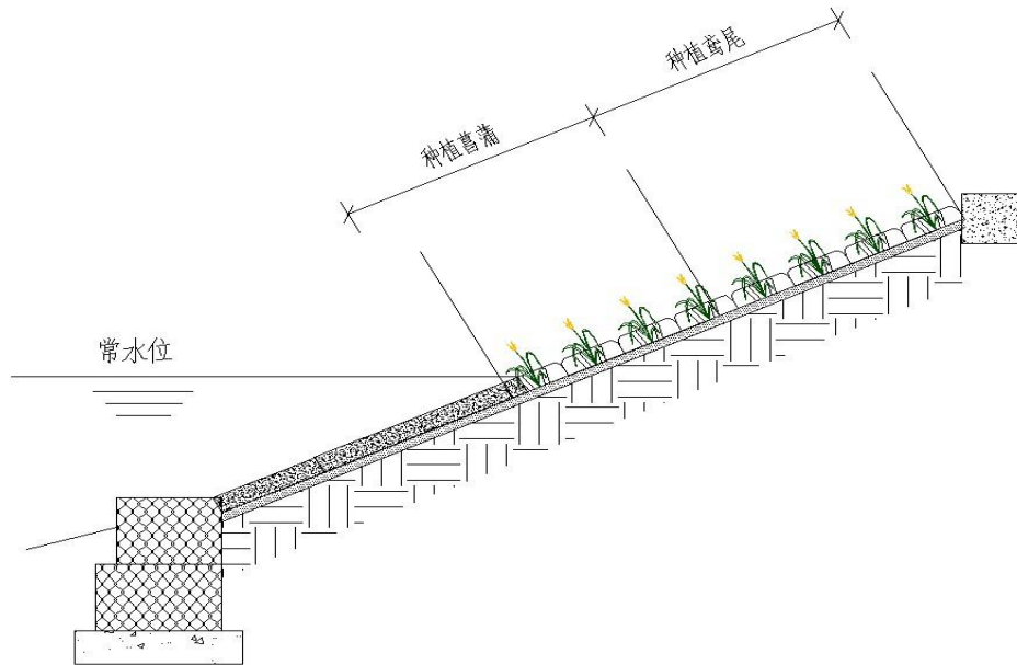
图 3.3-2 植物等比例种植示意图
