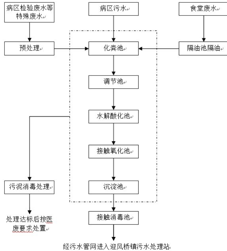
图 4-1 污水处理站处理工艺流程图
