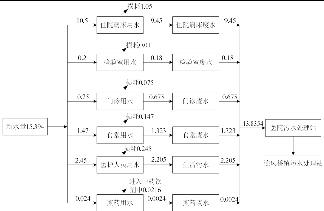
图 2-1 水平衡图 (单位: m 3 /d)
