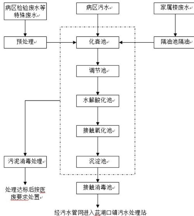
图 4-1 污水处理站处理工艺流程图
