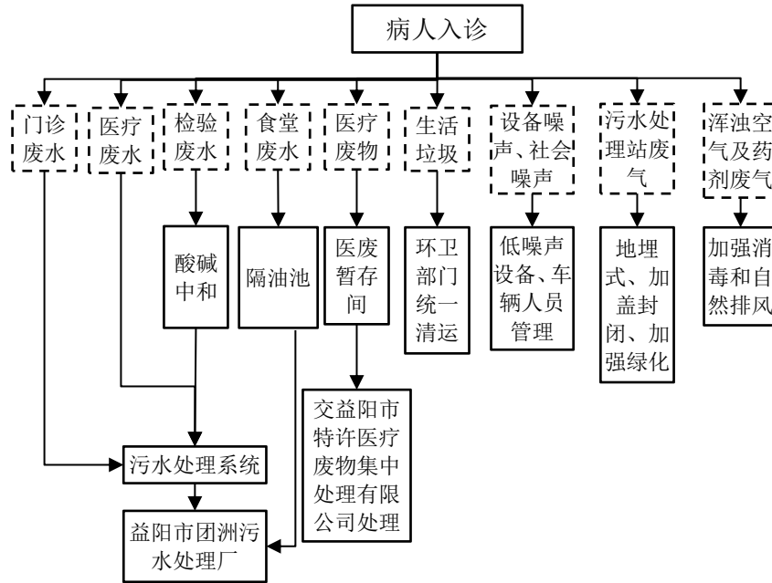
图 2-2 本项目运营期工艺流程及产污节点图
