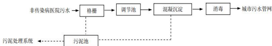
图 4-1 非传染病医院污水一级强化处理工艺流程
