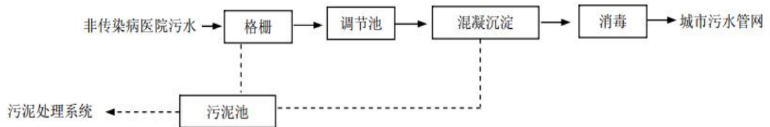
图 4-1 非传染病医院污水一级强化处理工艺流程
