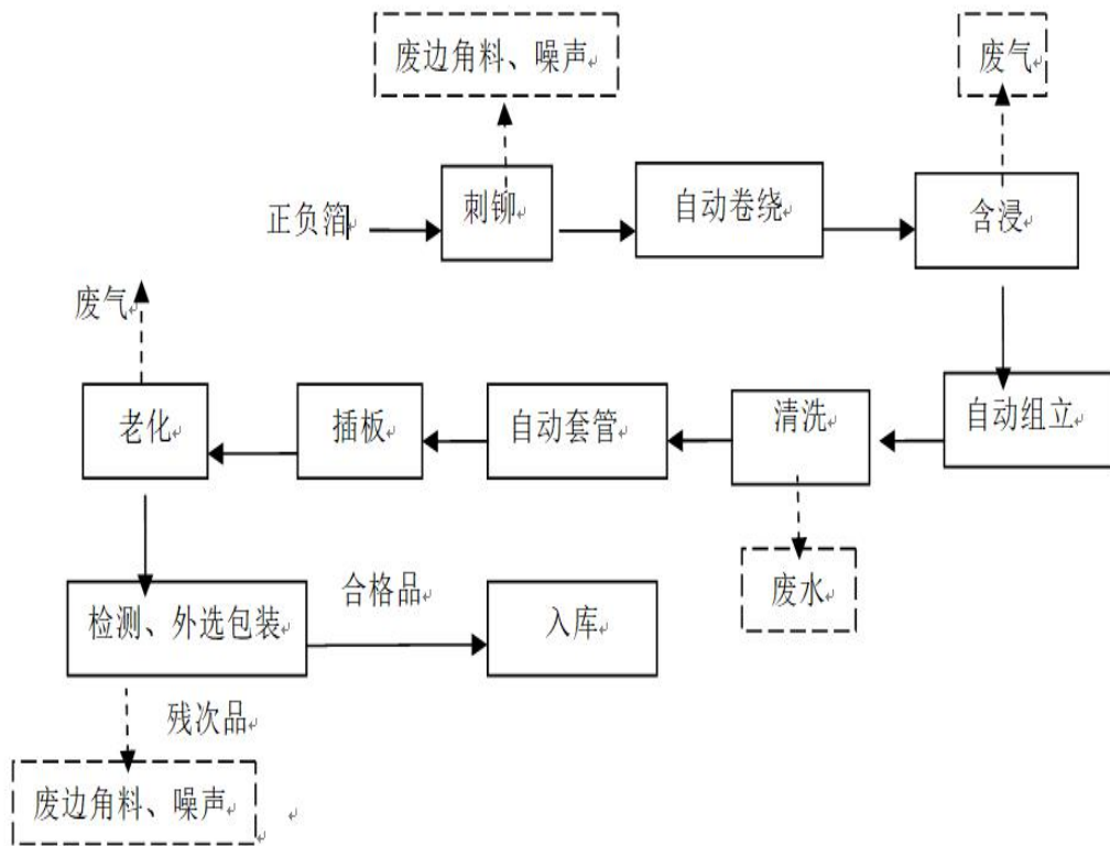
图 2-2 项目铝电解电容器生产工艺流程及产污节点图
