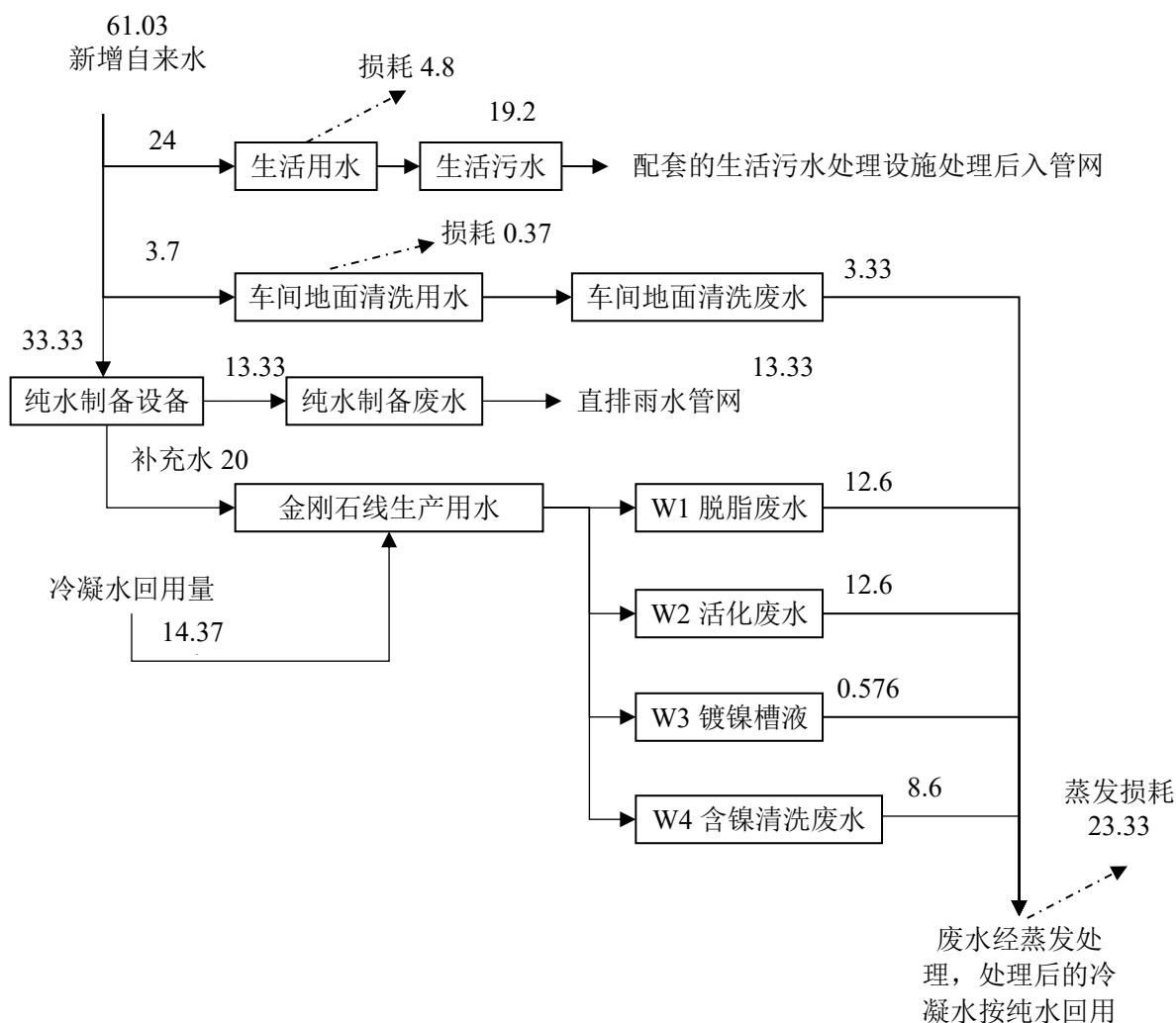
图3.4-3 项目水平衡图 单位: \text{m}^3/\text{d}
