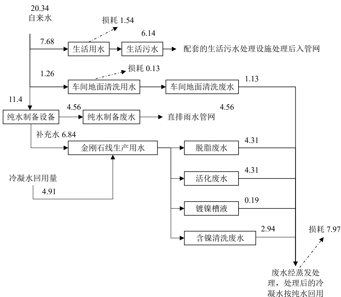
图3.1-1 现有工程给排水平衡图
