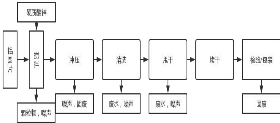
图 2-2 项目铝壳生产工艺流程及产污节点图
