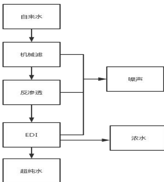
图 2-3 项目营运期纯水制备工艺流程图
