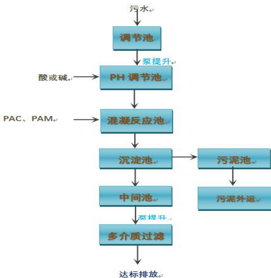
图 3-1 污水一体化设施工艺流程图
