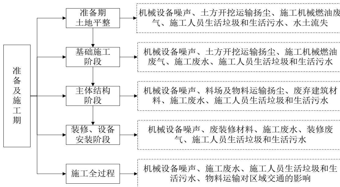
图 4-1 施工流程及产污节点示意图
