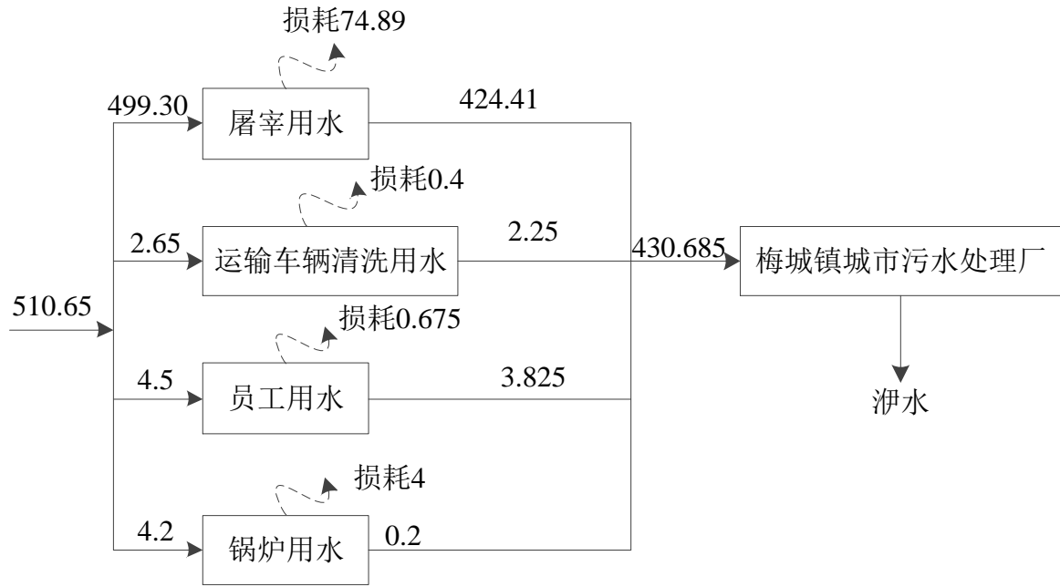
图 3-1 项目运营期水平衡分析图 (单位: m 3 /d)
