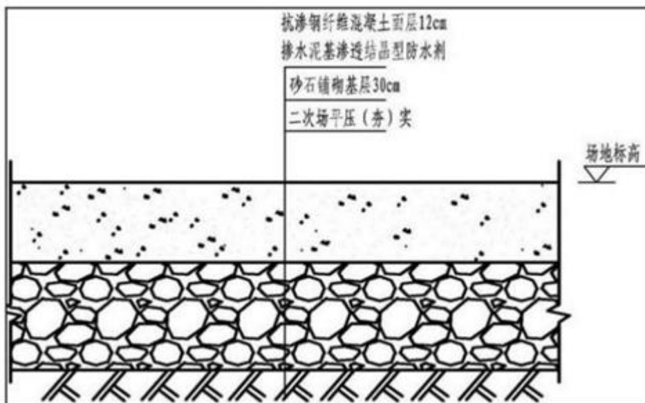
图 7-2 一般污染防渗区结构示意图
