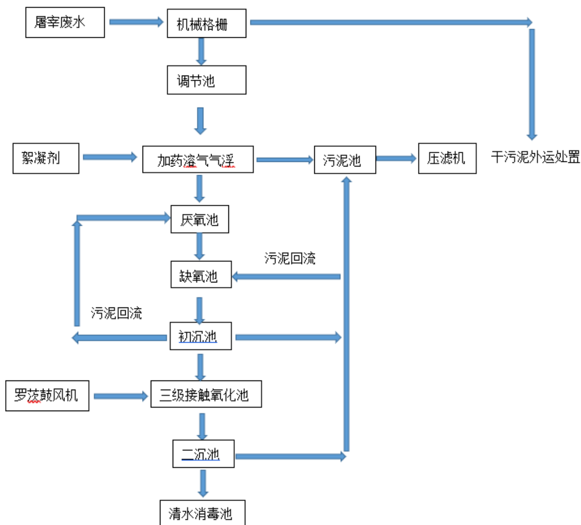
图 7-1 项目运营期污水处理工艺流程图
