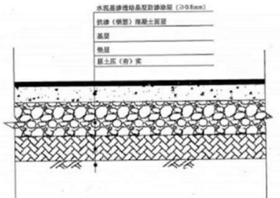
图 7-3 重点污染防渗区结构示意图
