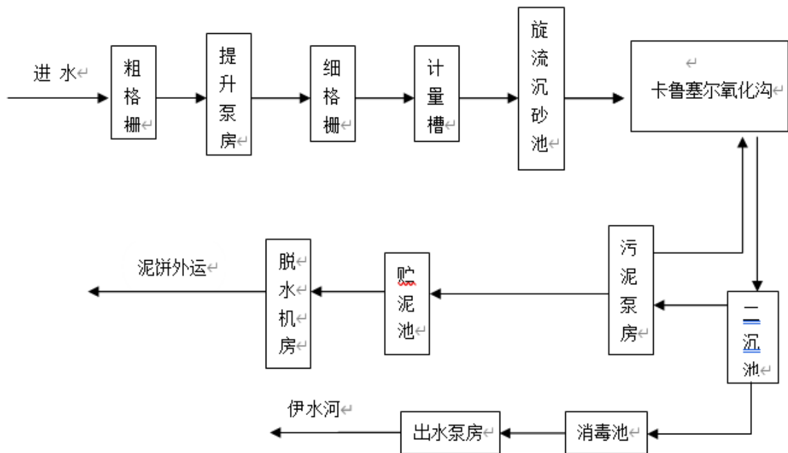
图 6-2 污水处理厂工艺图
