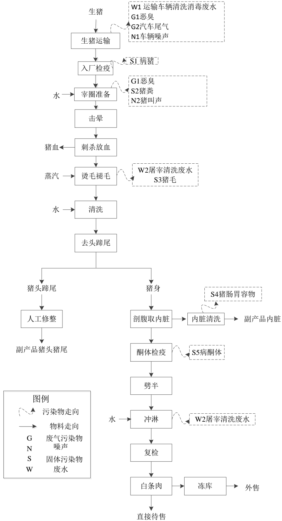
图 4-2 生猪屠宰工艺流程及产污环节图
