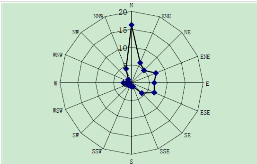
图 5-1 安化县历年全年风向玫瑰图
