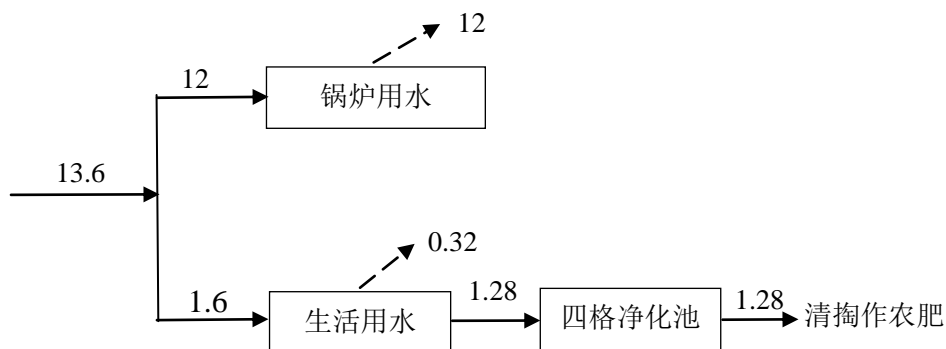
图2-1 项目水平衡图 (m³/d)
