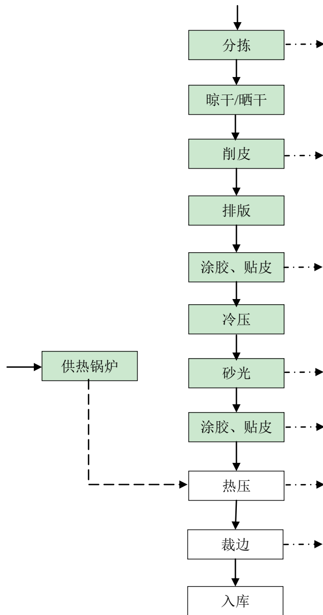
图 2-2 运营期生产工艺流程及产污环节图
