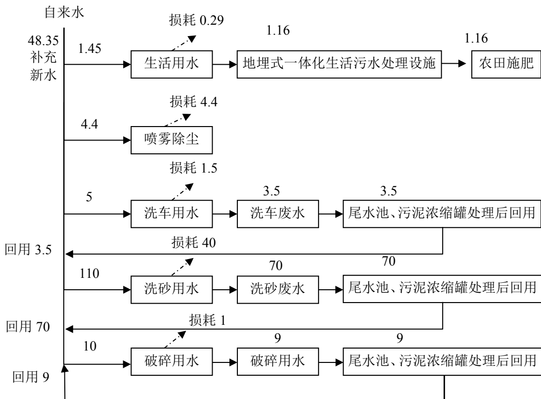
图 2-1 水平衡分析图 (m 3 /d)
