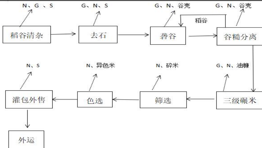
(注：G：废气 N：噪声 S：固废) 图 2-1 营运期工艺流程及产污节点图
