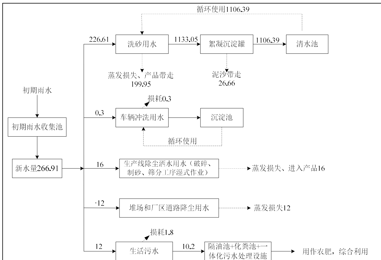
图 1-1 项目工程水平衡图 (单位: m^3/d )
