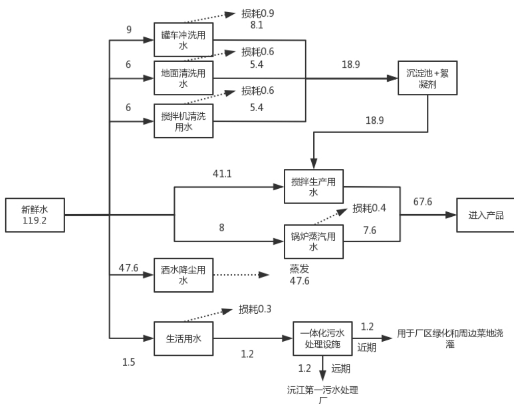
图 1-1 建设项目水平衡图（单位：m³/d）
