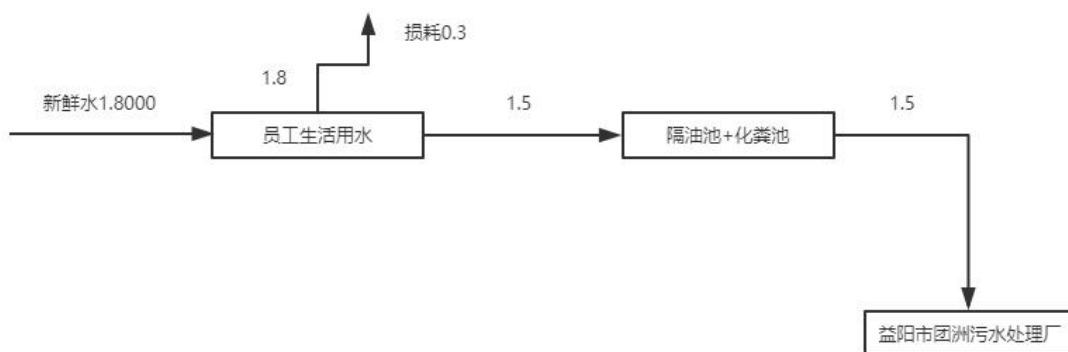
图 1-1 项目水平衡图 (t/d)
