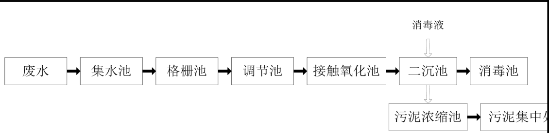
图 7-1 污水处理站工艺流程图
