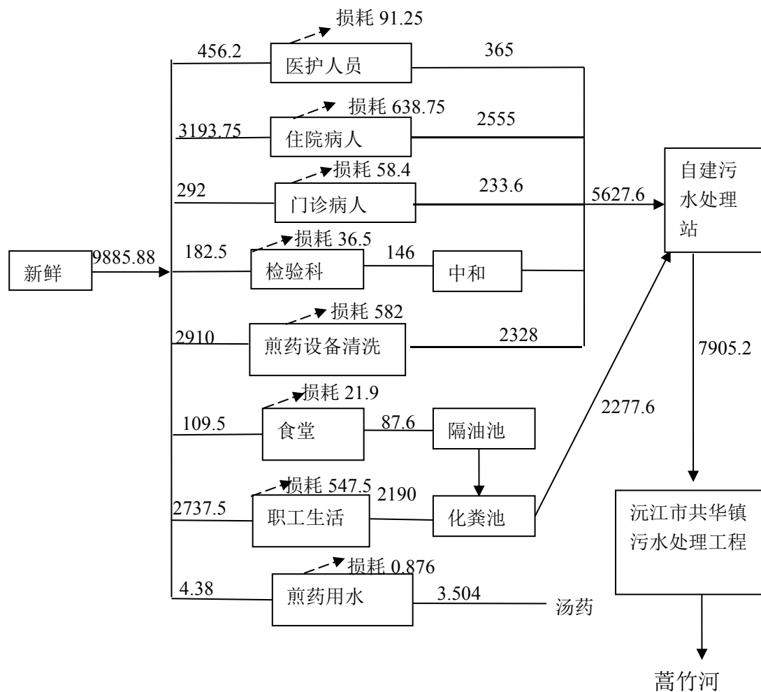
图 1-1 项目水平衡图单位：m³/a
