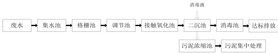
图 7-1 一体化污水处理站工艺流程图
