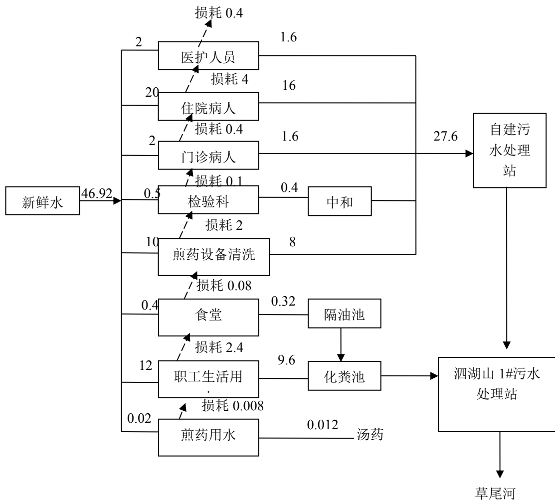
图 1-1 项目水平衡图单位: m 3 /d
