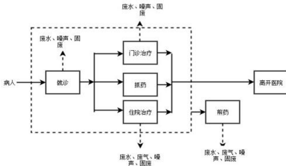
图 5-1 项目营运期工作流程及产污节点图
