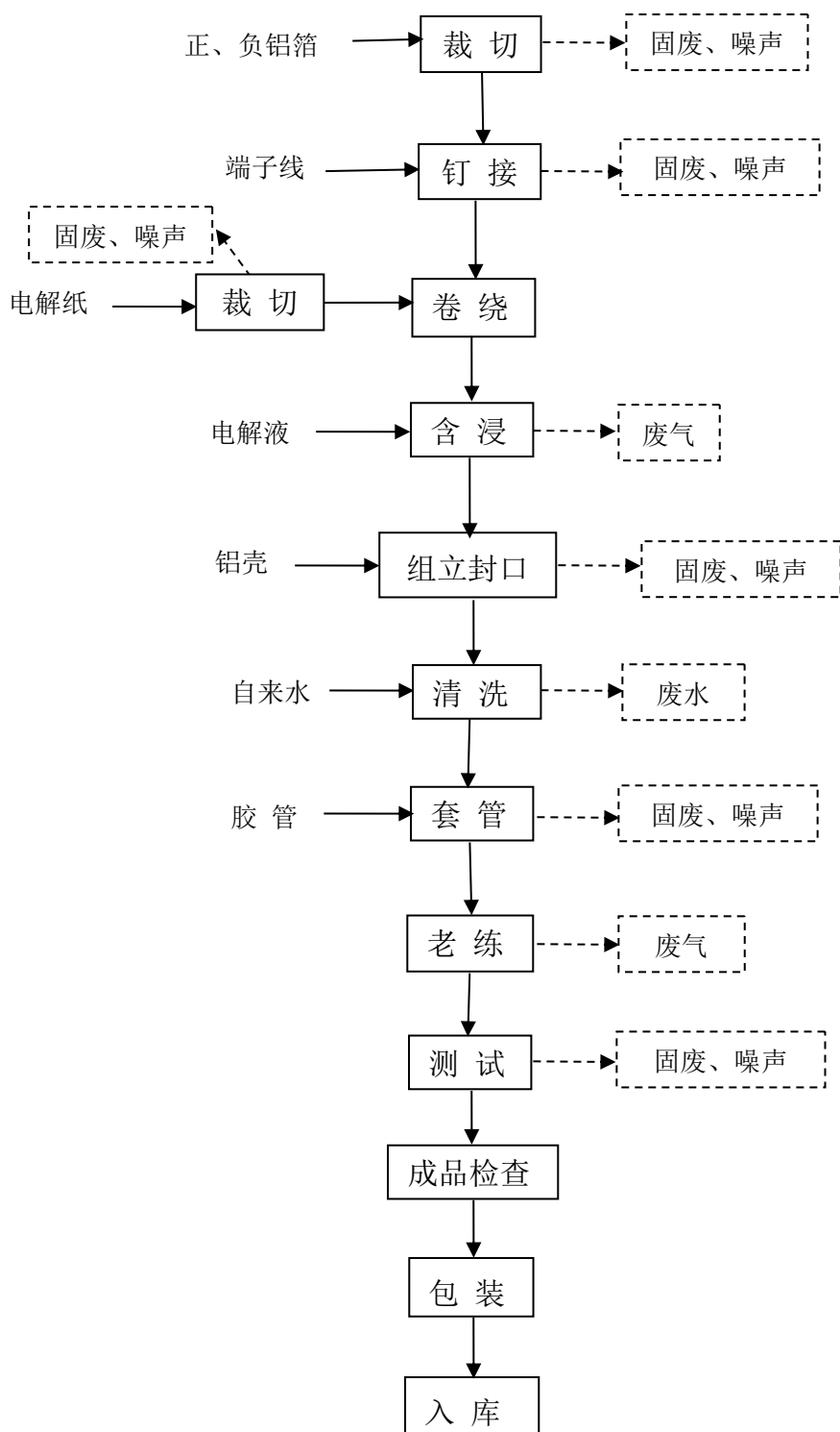
图 4-1 电解电容器生产工艺流程及产污环节图
